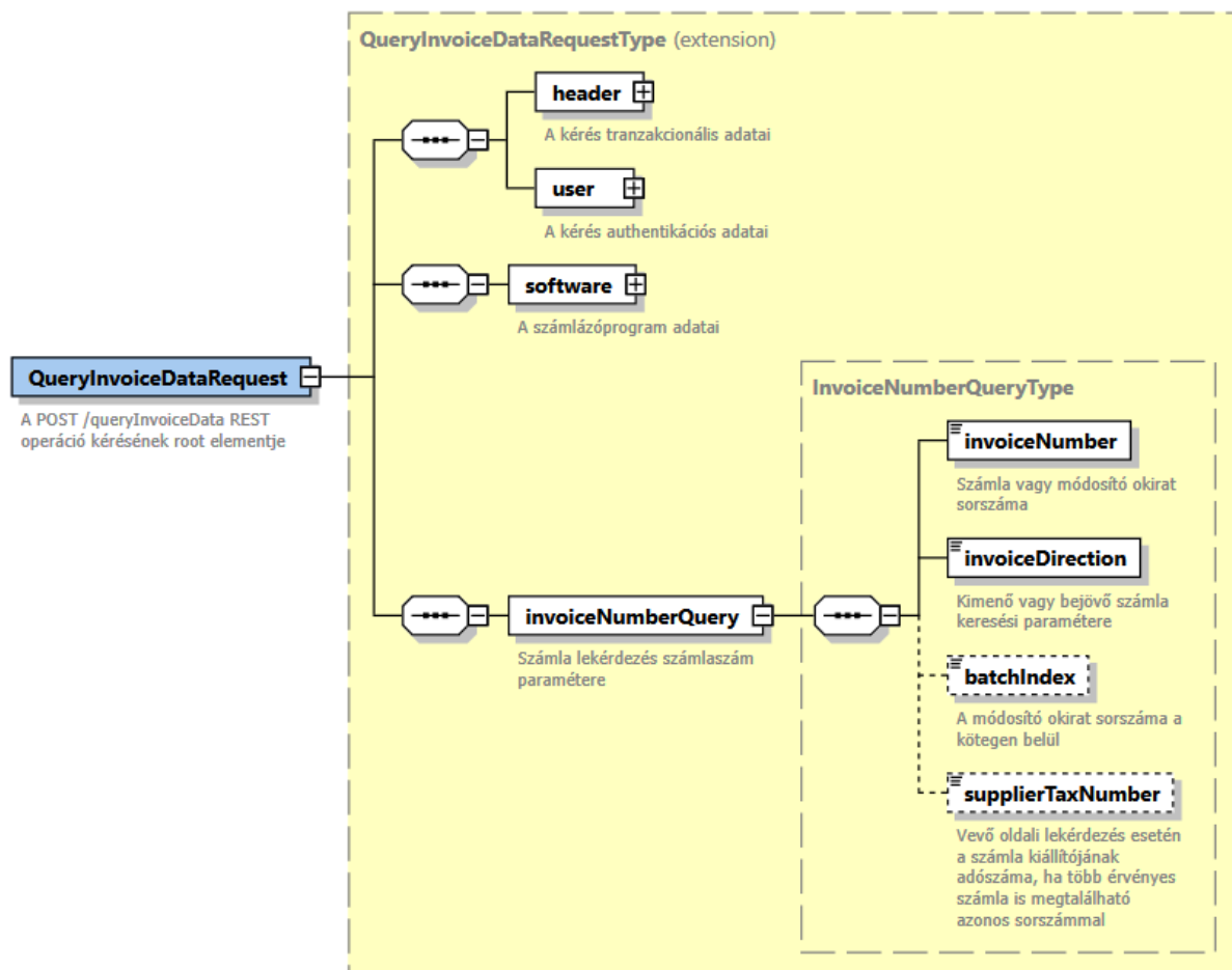
16. ábra A QueryInvoiceDataRequest felépítése
