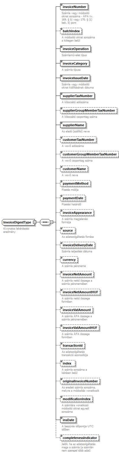
25. ábra Az InvoiceDigestType felépítése
