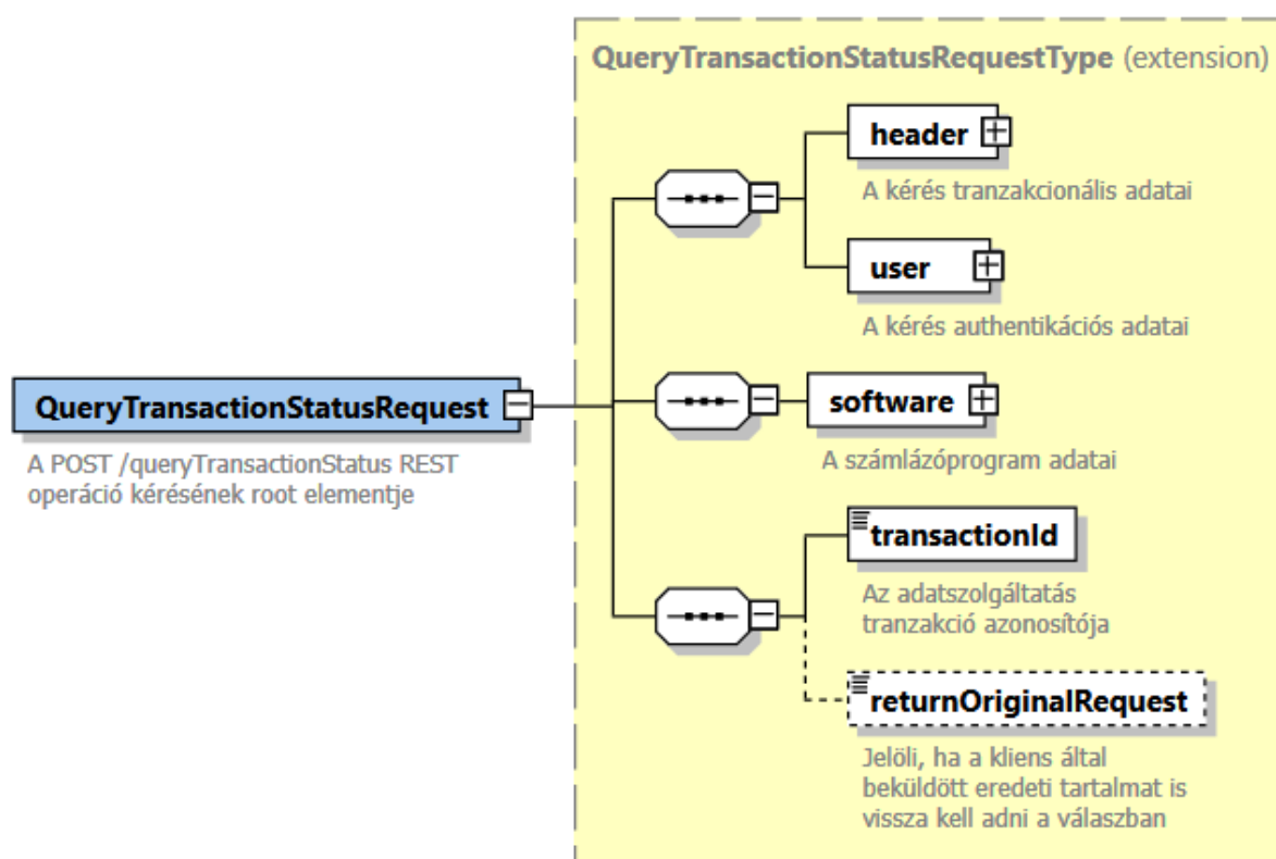
28. ábra A QueryTransactionStatusRequest felépítése
